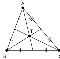
(d) Centroid
